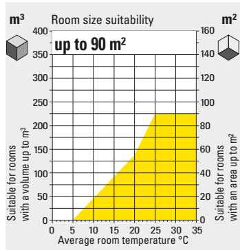
TTK 90 E
