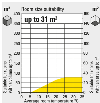
TTK 52 E
